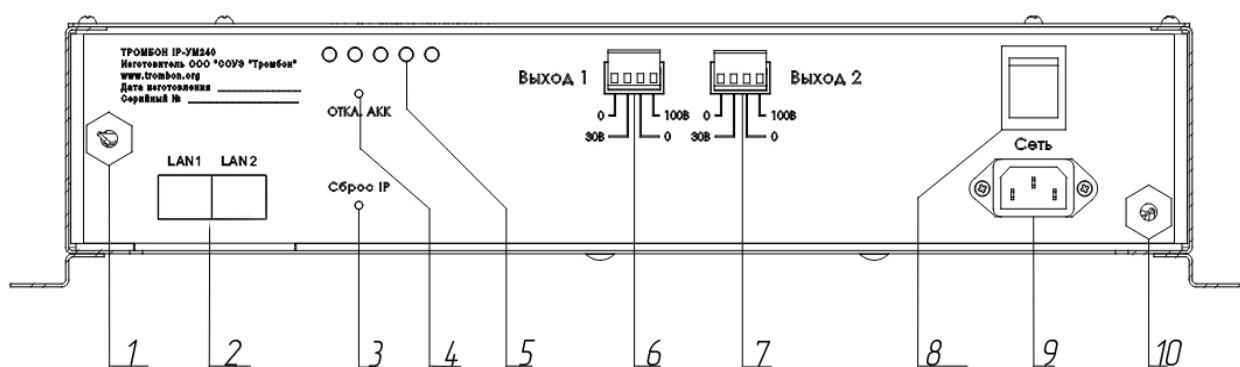
Рисунок 3 - Коммутационный отсек, вид снизу
