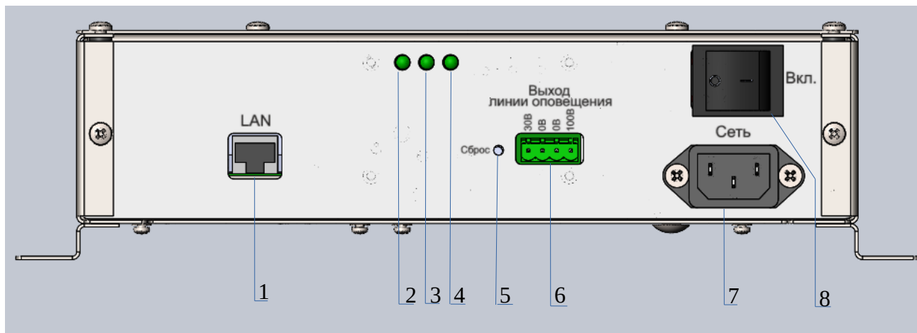
Рисунок 2 - Коммутационный отсек, вид снизу
